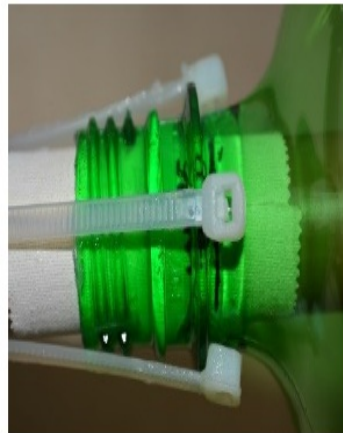
Fig. 17. Posição das cabeças das abraçadeiras sobre o anel sustentação.
