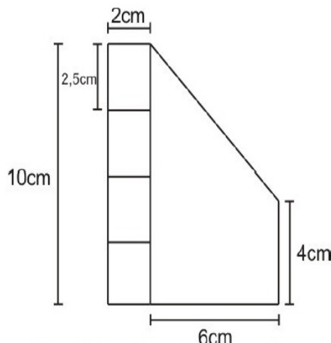
Fig. 2. Dimensões e formato da aleta
